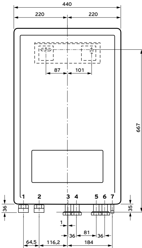
Mindestabstände und Montagefreiräume
