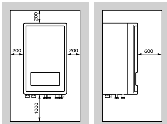
Mindestabstände und Montagefreiräume
