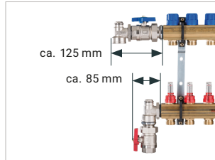
Verteiler-Anschluss-Set 90° (Art.-Nr. 291100)
