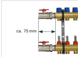
Verteiler-Anschluss-Set Durchgang (Art.-Nr. 295100)
