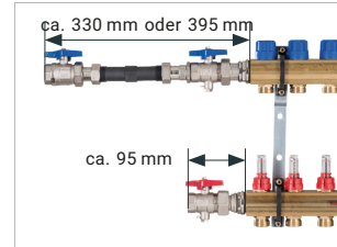
WMZ-Anschluss-Set Durchgang (Art.-Nr. 721017 oder 721027)
