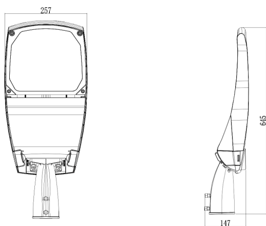
Maßskizze
