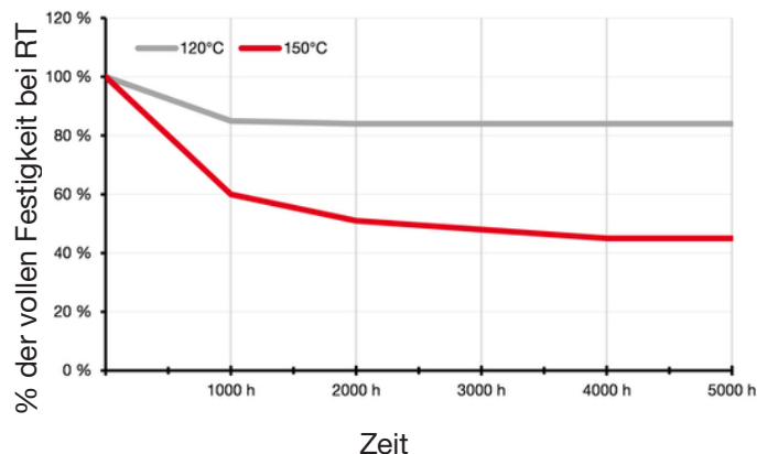
Wärmealterung
