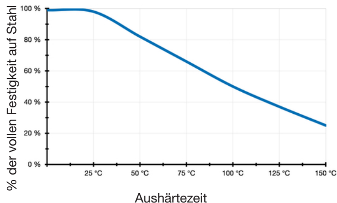
Reaktionsgeschwindigkeit bei unterschiedlichen Temperaturen
