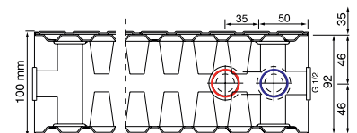
Typ 22 links Bautiefe 100 mm
