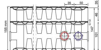
Typ 33 links Bautiefe 155 mm
