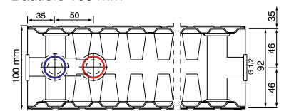
Typ 33 rechts Bautiefe 155 mm
