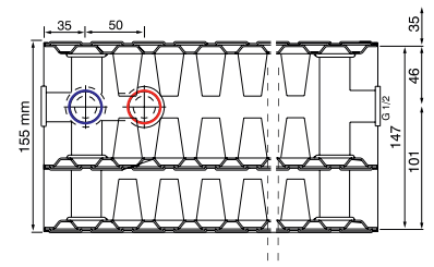
Typ 33 links Bautiefe 155 mm
